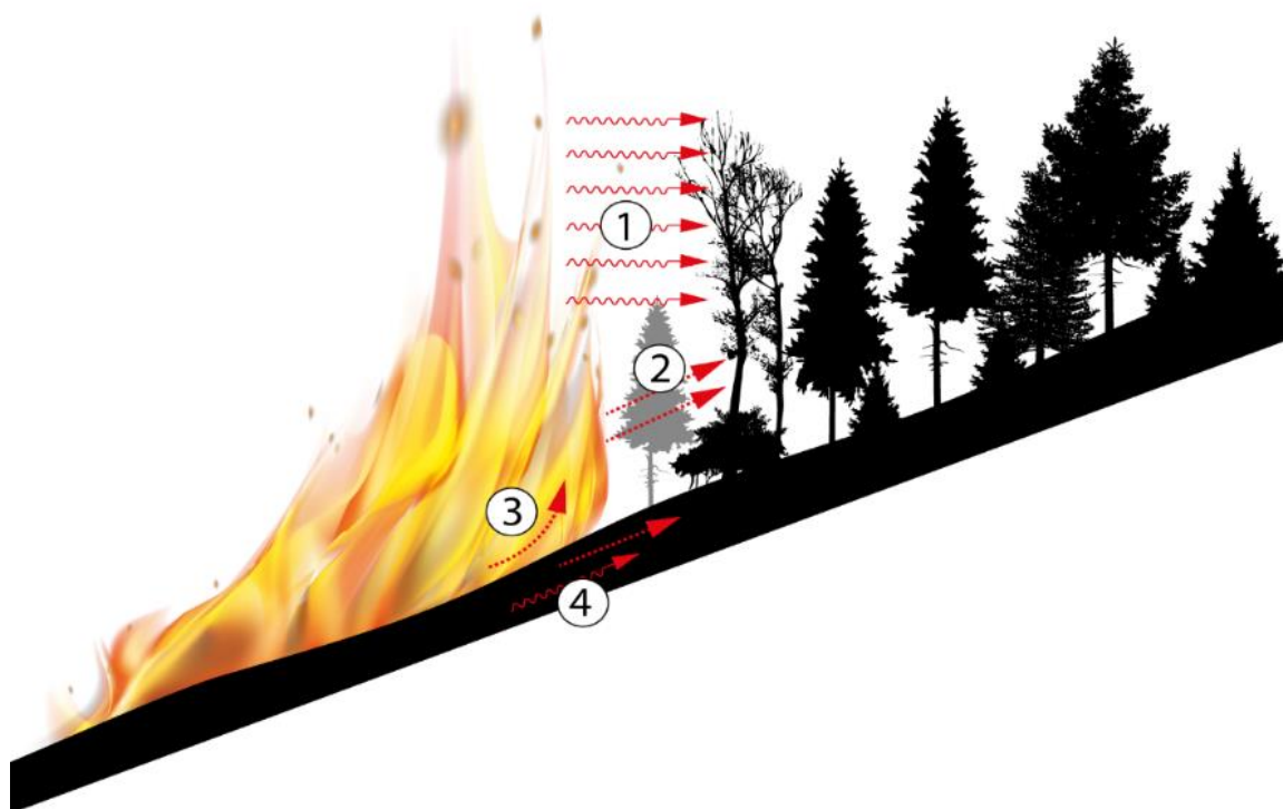
Obr. 6 - Přenos tepla fronty požáru ve svahovitém terénu
