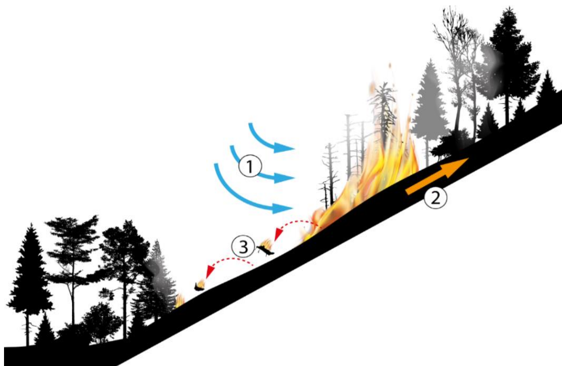
Obr. 7 - Šíření lesního požáru směrem dolů ve svahovitém terénu
